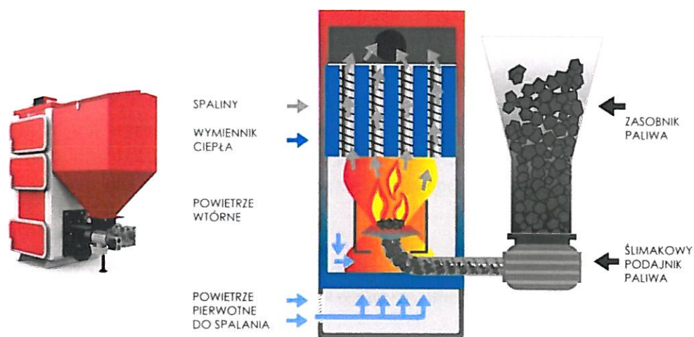
Rysunek 1. Przekrój nowoczesnego kotła retortowego
